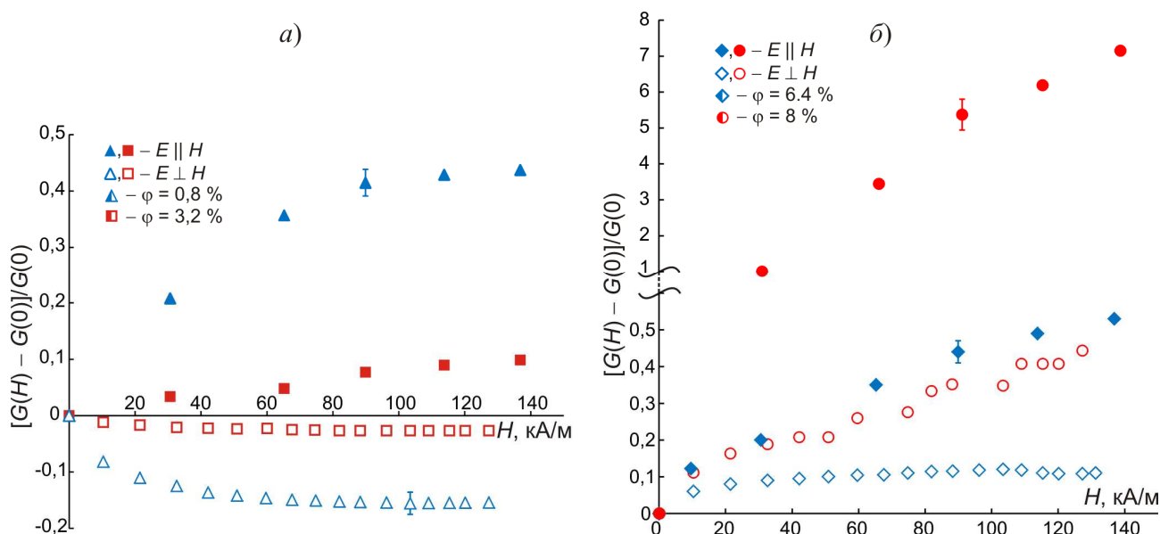
Рис. 2. Зависимости относительного изменения проводимости ячейки от величины напряженности внешнего магнитного поля при различных взаимных ориентация магнитного и электрического полей: а – при низких концентрациях графита; б – при высоких концентрациях графита
