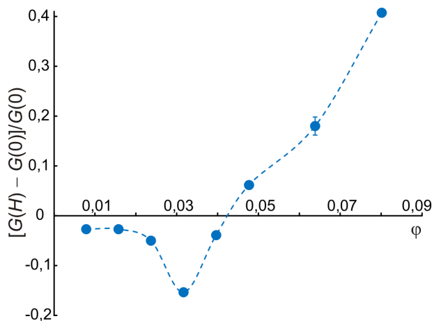
Рис. 5. Концентрационная зависимость относительного изменения проводимости ячейки, вызванного действием магнитного поля H = 88 кА/м, направленного перпендикулярно измерительному электрическому полю
