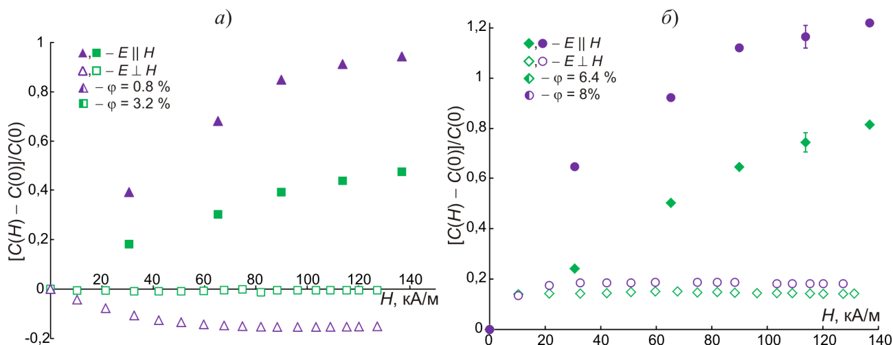
Рис. 3. Зависимости относительного изменения емкости ячейки от величины напряженности внешнего магнитного поля при различных взаимных ориентация магнитного и электрического полей: а – при низких концентрациях графита; б – при высоких концентрациях графита
