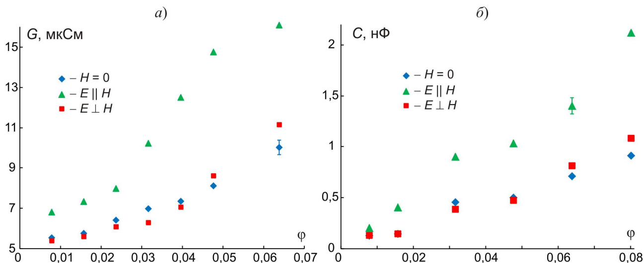
Рис. 4. Зависимости проводимости ( а ) и емкости ( б ) ячейки от объемной концентрации графита в отсутствии магнитного поля, в параллельных электрическом и магнитном полях ( H = 230 кА/м), а также в перпендикулярных электрическом и магнитном полях ( H = 88 кА/м)
